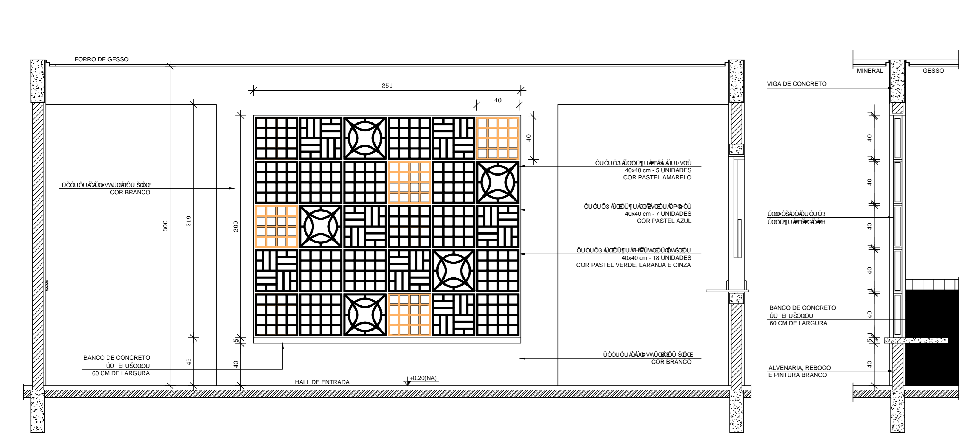
3 DETALHE 01 ESCALA 1/25
