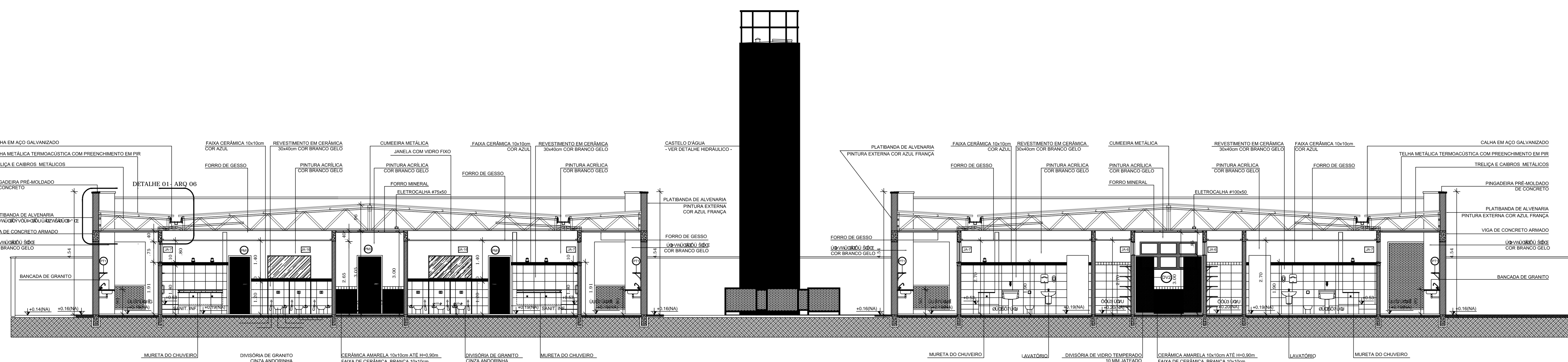
2 CORTE EE ESCALA 1/75
