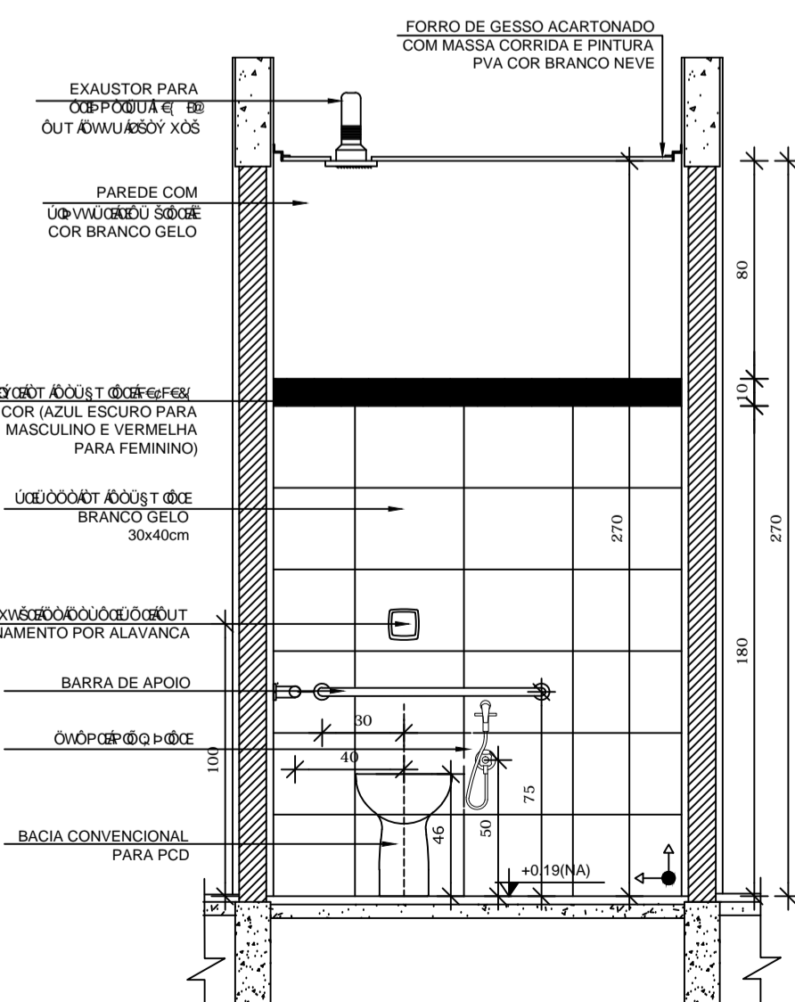
VISTA 7
