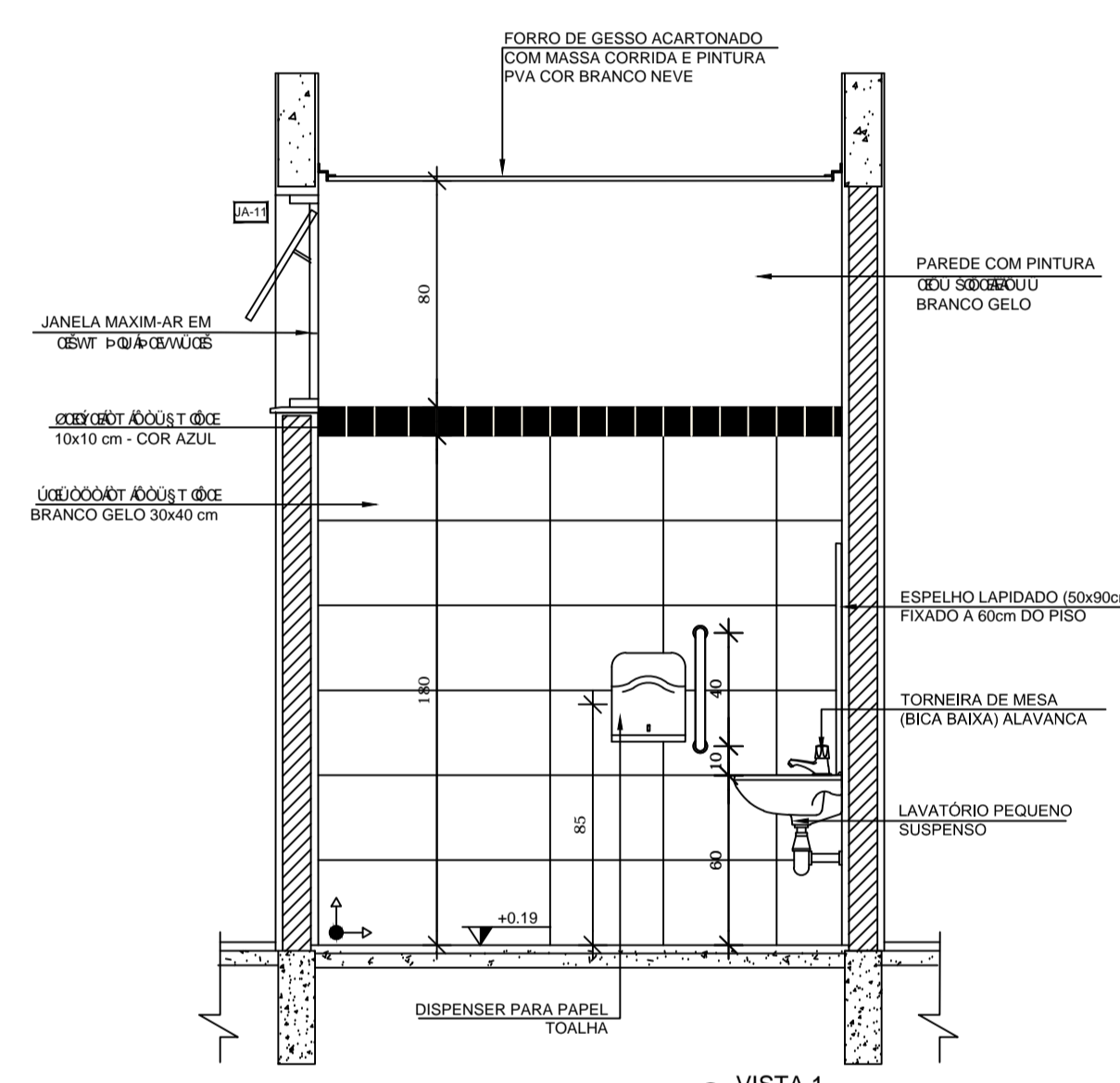
VISTA 1
