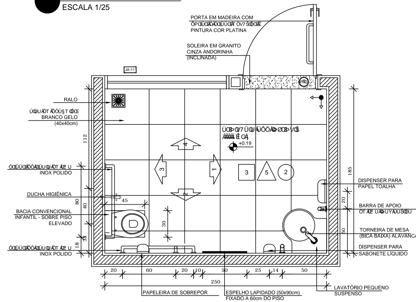
PLANTA BAIXA
