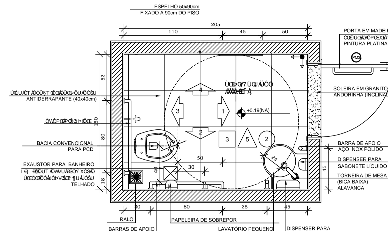
PLANTA BAIXA
